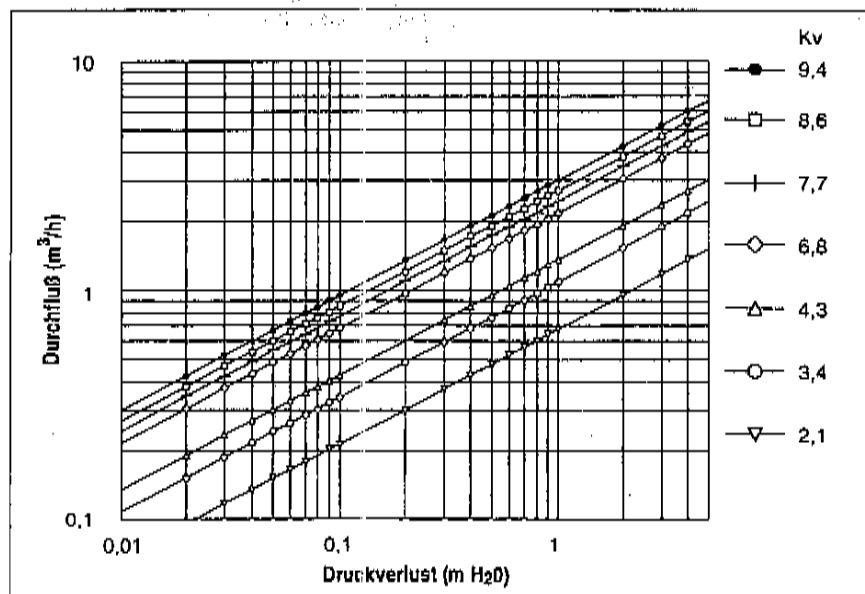
Bild 6 Druckabfall-Charakteristik
