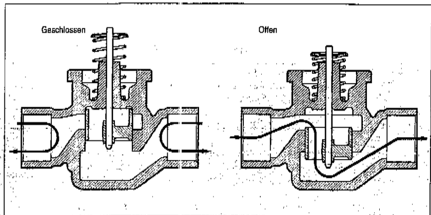
Bild 1 Zweiwege-Ventil
