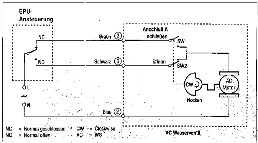
Bild 3 Anschlußplan für Antrieb mit EPU-Ansteuerungen
