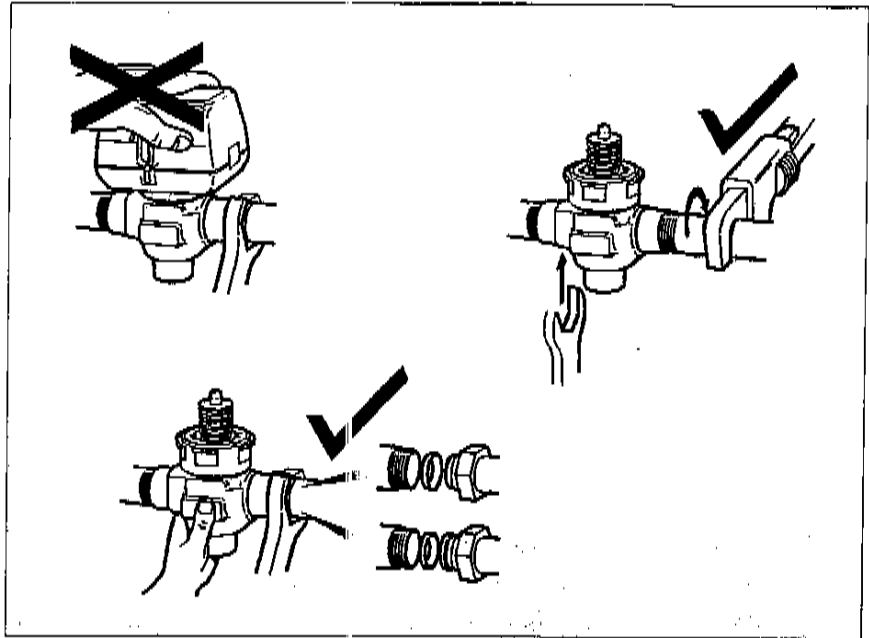
Bild 9 Installation
