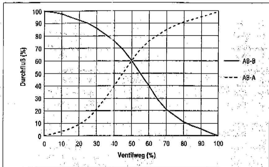
Bild 5 Durchfluß-Charakteristik eines Dreiwege-Ventils bei konstantem Druck an Anschluß AB
