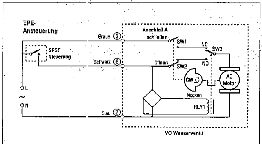
Bild 4 Anschlußplan für Antrieb mit EPE-Ansteuerungen
