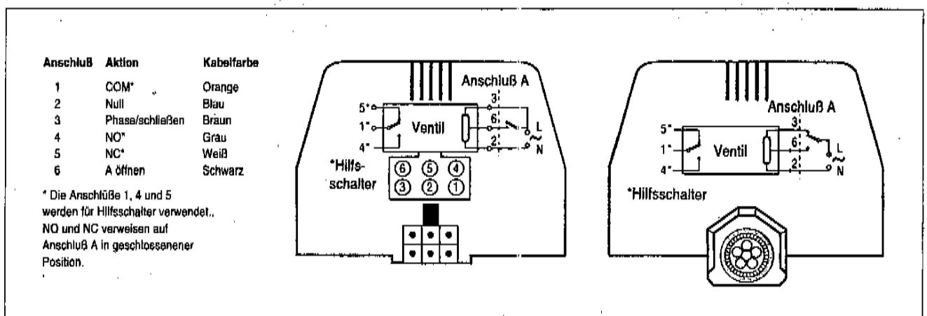
Bild 8 Anschluß-Farben
