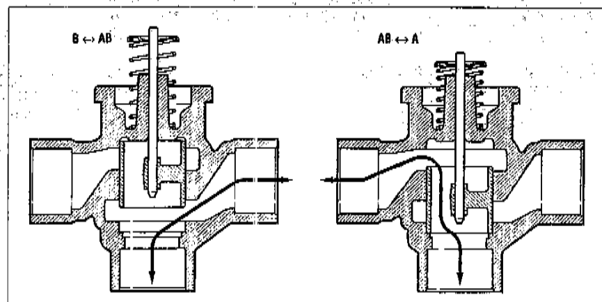
Bild 2 Dreiwege-Ventil
